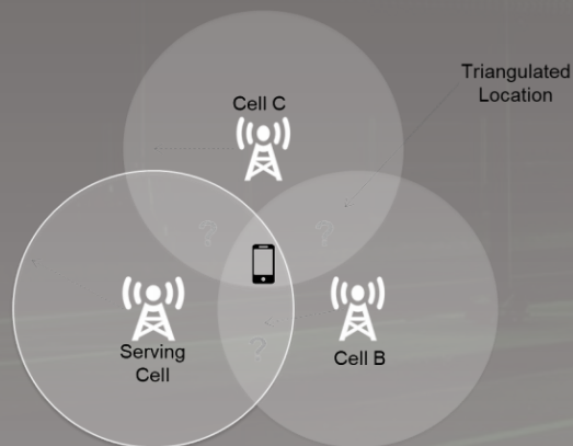
三角定位法
