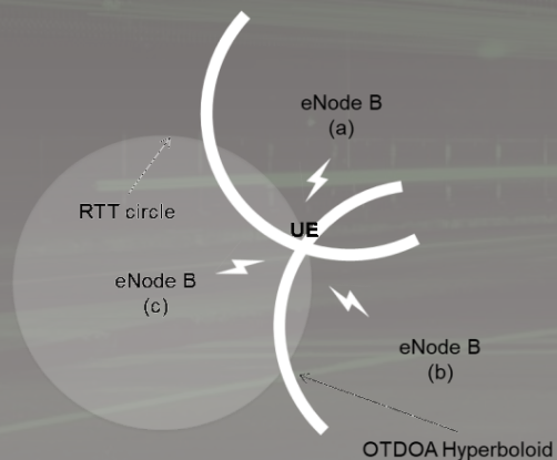
多點定位法
